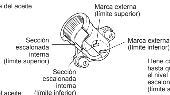
Fig. 2 Conducto del aceite
